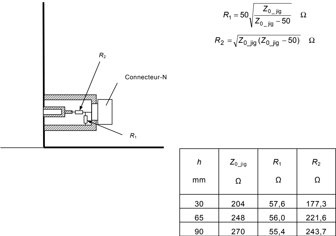
Figure 24 – Exemple d'un adaptateur d'impédance avec réseau résistif
